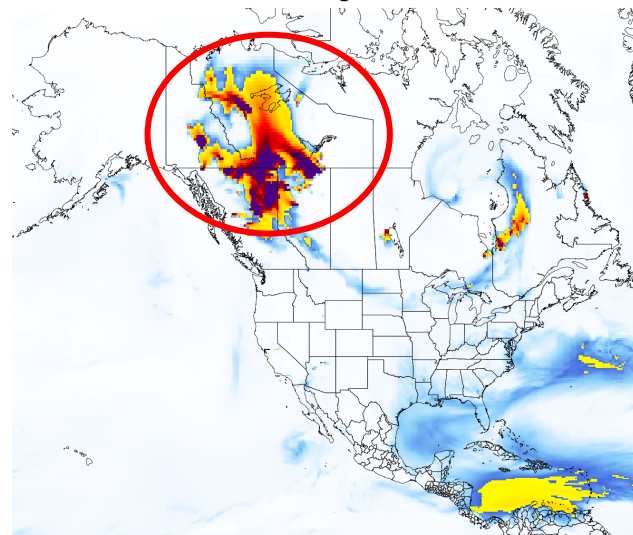
NAAPS PM_{2.5}
