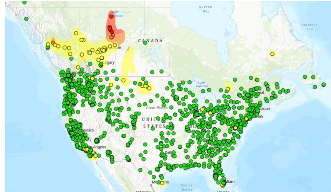
AirNow AQ
