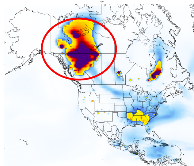
NAAPS PM_{2.5}
