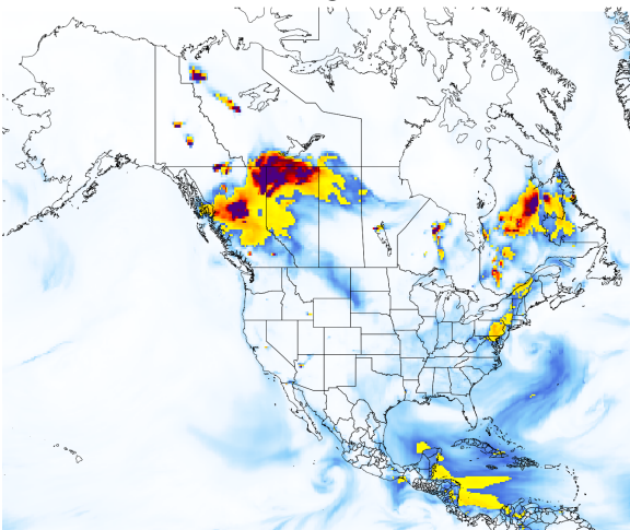
GEOS-FP PM_{2.5}
