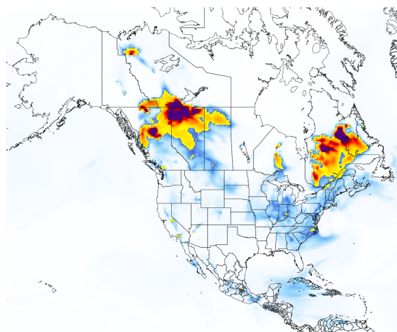
GEOS-CF PM_{2.5}
