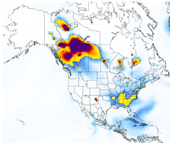
NAAPS PM_{2.5}
