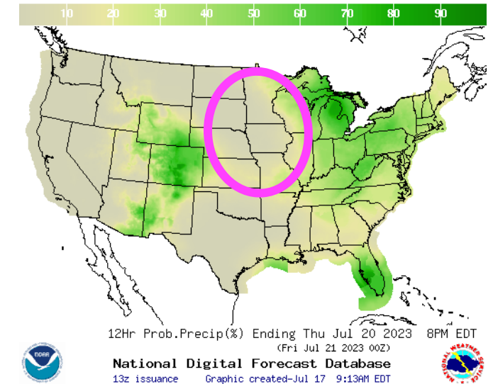
Precip Prob.
