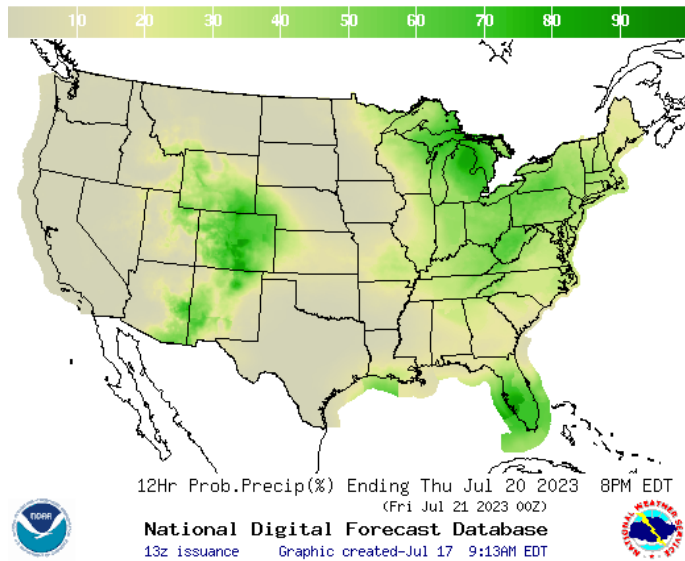
Precip Prob.
