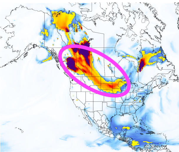
GEOS-FP \text{PM}_{2.5}
