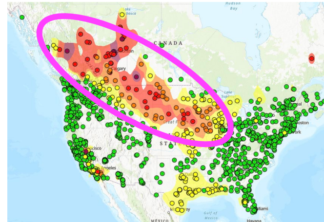
AirNow AQ
