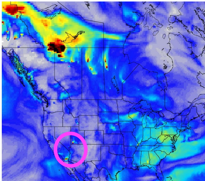
GEOS-FP
