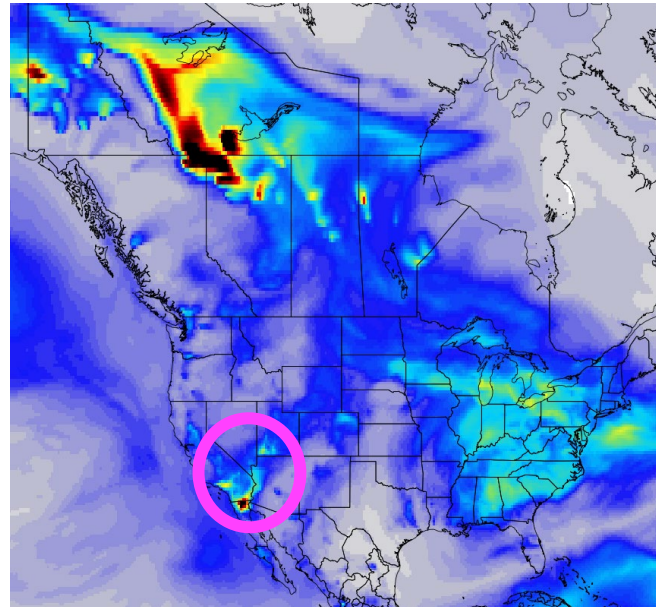
GEOS-CF
